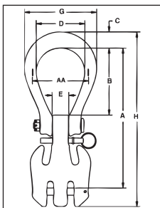
A-1362 Crosby ELIMINATOR® Gancho Doble
