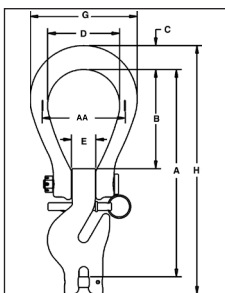
A-1361 Crosby ELIMINATOR® Gancho Único
